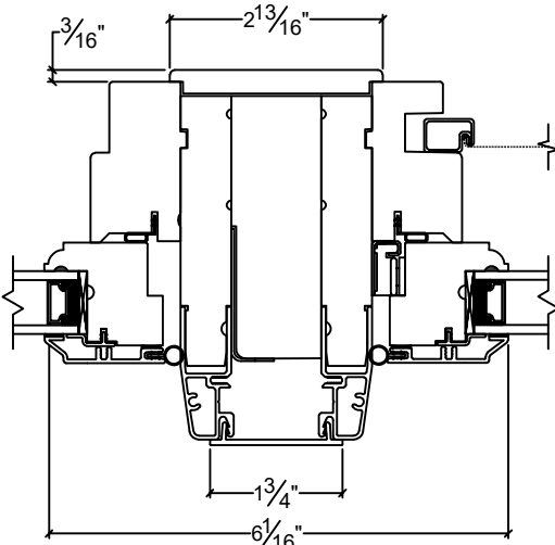
Transom & Casement Clad Mull 3 1/2" Jamb c/w 1 3/16" Filler
