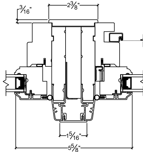
Transom & Casement Clad Mull 3 1/2" Jamb c/w 3/4" Filler
