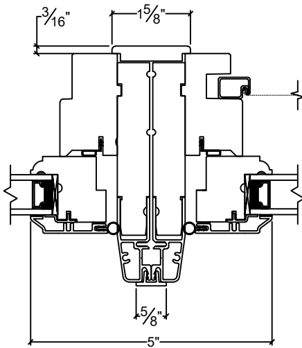
Transom & Casement Clad Mull 3 1/2" Jamb
