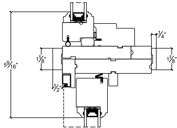
TRANSOM / DH500 STACK 4 9/16" JAMB
