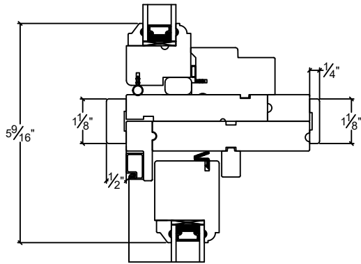
TRANSOM / DH500 STACK 4 9/16" JAMB
