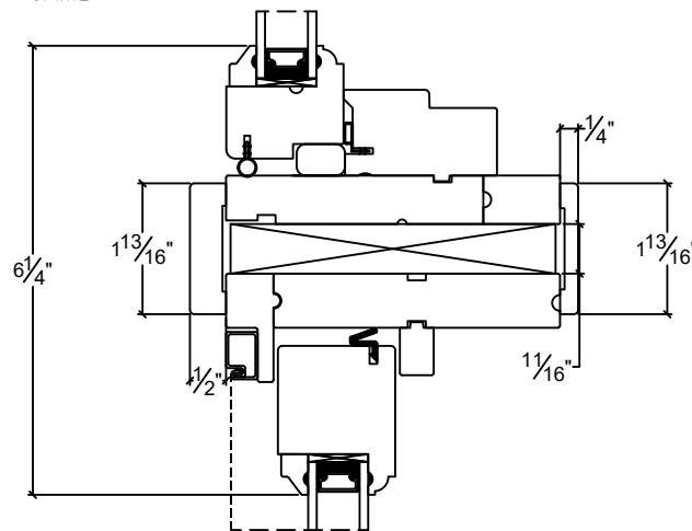
TRANSOM / DH500 STACK 4 9/16" JAMB C/W FILLER
