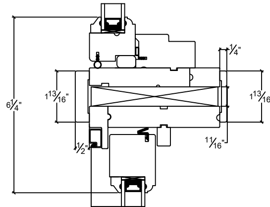
TRANSOM / DH500 STACK 4 9/16" JAMB C/W FILLER
