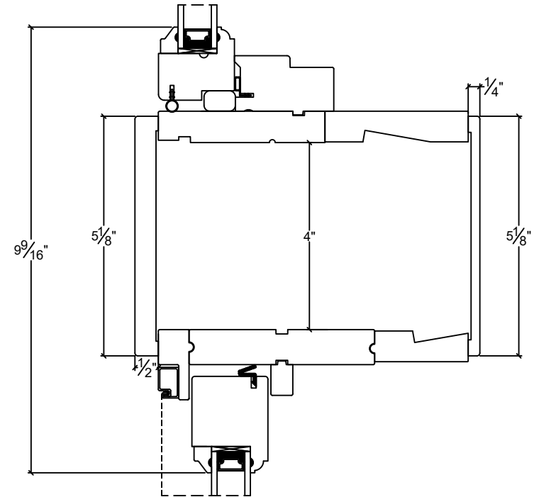
TRANSOM / DH500 STACK 6 9/16" JAMB C/W POCKET
