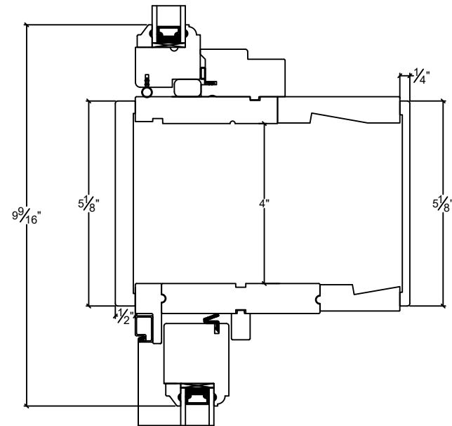
TRANSOM / DH500 STACK 6 9/16" JAMB C/W POCKET
