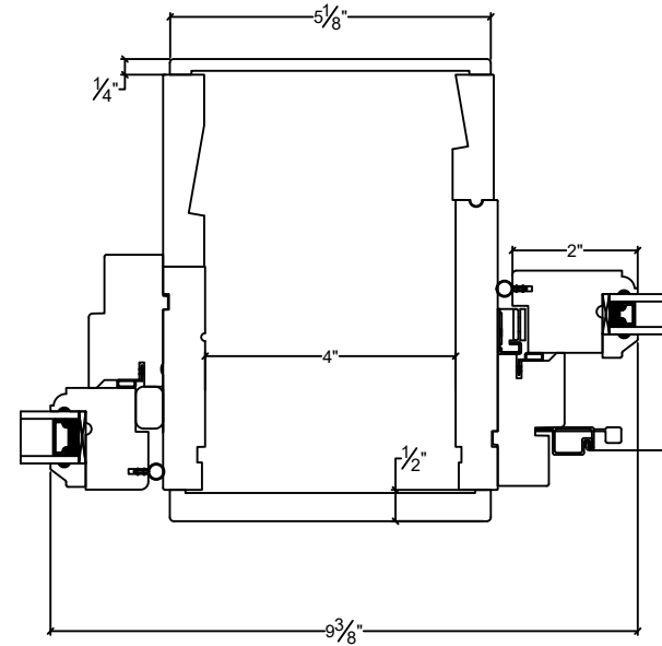
TRANSOM / HOPPER MULL 6 9/16" JAMB C/W POCKET
