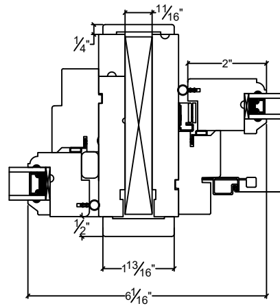
TRANSOM / HOPPER MULL 4 9/16" JAMB C/W FILLER
