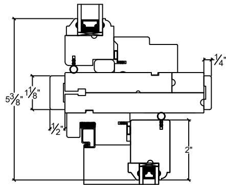
TRANSOM / HOPPER STACK 4 9/16" JAMB
