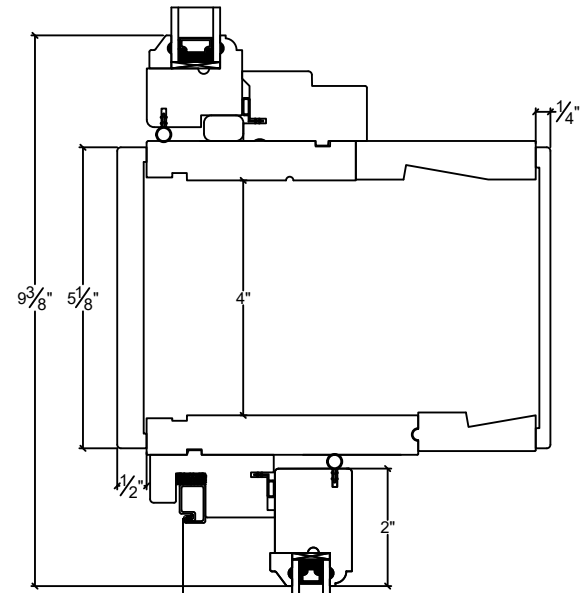
TRANSOM / HOPPER STACK 6 9/16" JAMB C/W POCKET
