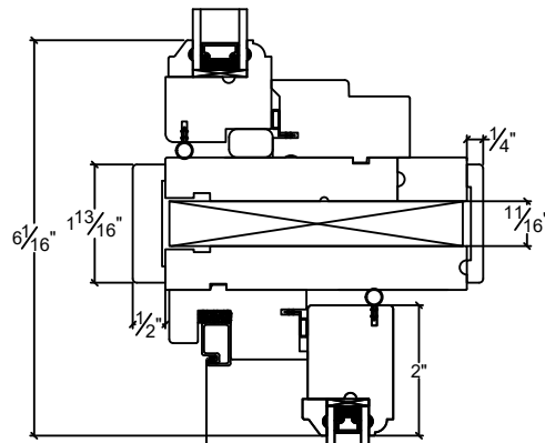
TRANSOM / HOPPER STACK 4 9/16" JAMB C/W FILLER
