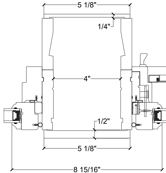
TRANSOM / AWNING MULL 6 9/16" JAMB C/W POCKET
