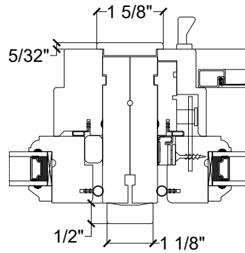
TRANSOM / AWNING MULL 3 1/2" JAMB
