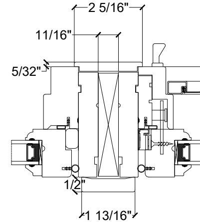
TRANSOM / AWNING MULL 3 1/2" JAMB C/W FILLER
