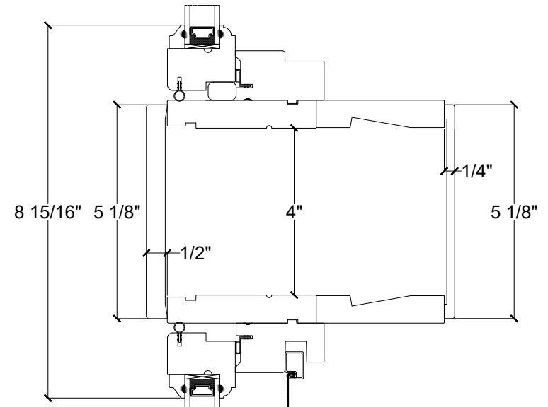
TRANSOM / AWNING STACK 6 9/16" JAMB C/W POCKET
