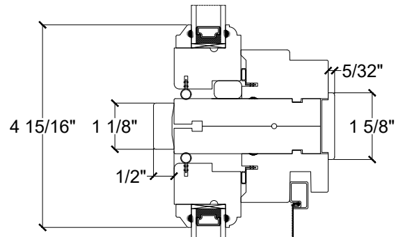
TRANSOM / AWNING STACK 3 1/2" JAMB
