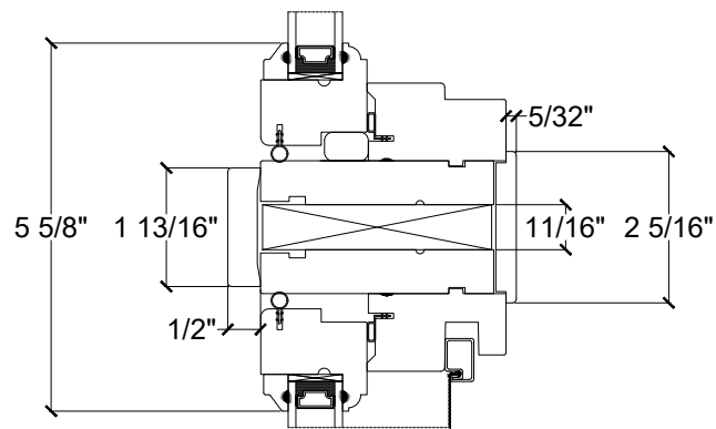
TRANSOM / AWNING STACK 3 1/2" JAMB C/W FILLER
