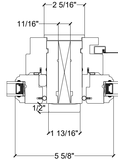
TRANSOM / CASEMENT MULL 3 1/2" JAMB C/W FILLER
