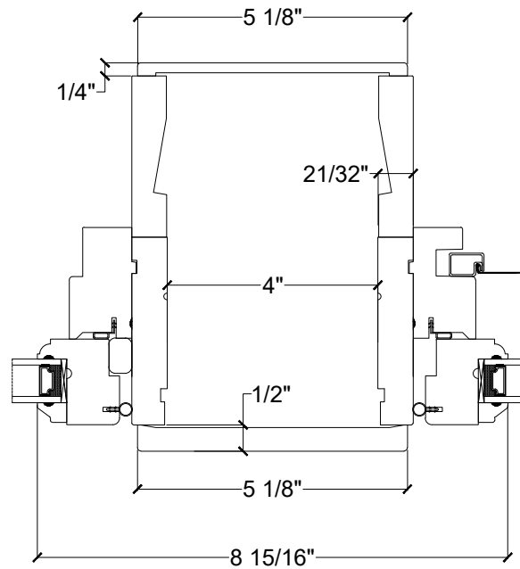
TRANSOM / CASEMENT MULL 6 9/16" JAMB C/W POCKET
