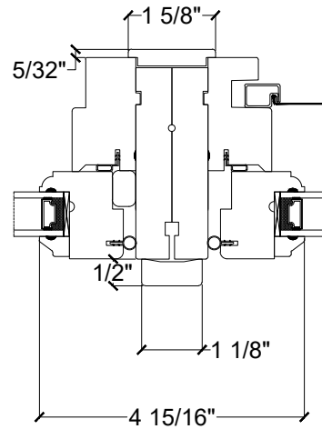
CASEMENT MULL 3 1/2" JAMB
