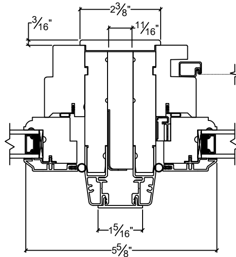
Transom & Casement Clad Mull 3 1/2" Jamb c/w 11/16" Filler
