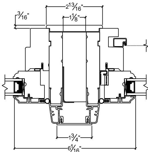
Transom & Casement Clad Mull 3 1/2" Jamb c/w 1 1/8" Filler
